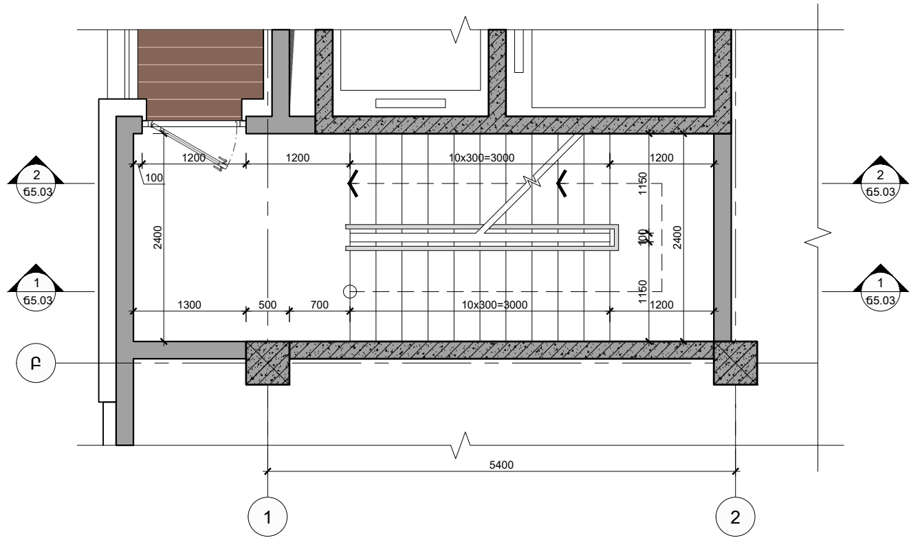
ԱՍՏԻՃԱՆԱՎԱՆՂԱԿ 1, ԴՐՎԱԳ 3 (3,4,5,6,7-ՐԴ ՀԱՐԿԵՐԻ ՀԱՏԱԿԱԳԻԾ) Մ 1:50
