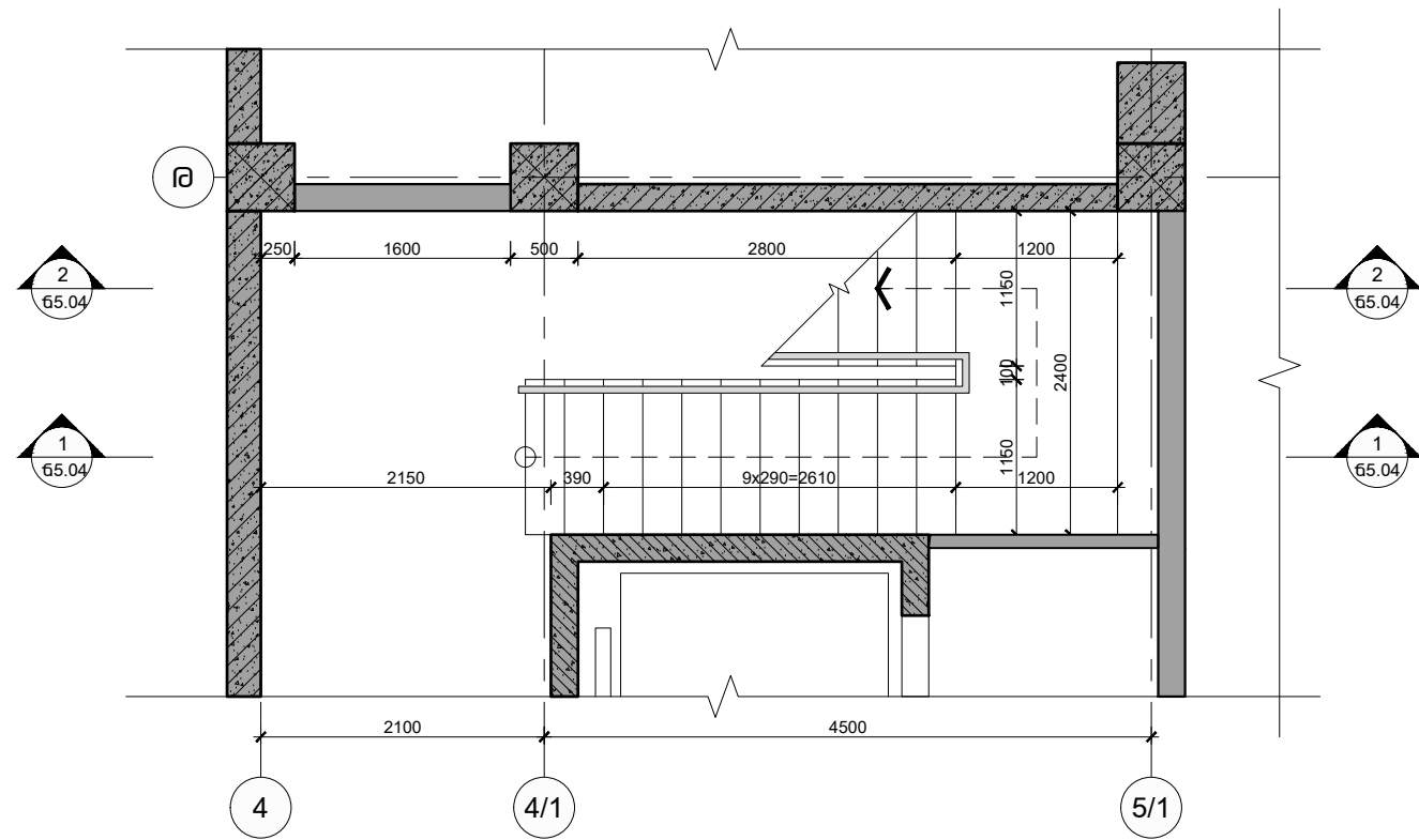
ԱՍՏԻՃԱՆԱՎԱՆՂԱԿ 2, ԴՐՎԱԳ 3 (3,4,5,6,7-ՐԴ ՀԱՐԿԵՐԻ ՀԱՏԱԿԱԳԻԾ) Մ 1:50
