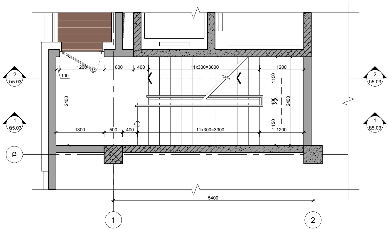
ԱՍՏԻՃԱՆԱՎԱՆՂԱԿ 1, ԴՐՎԱԳ 4 (8-ՐԴ ՀԱՐԿԻ ՀԱՏԱԿԱԳԻԾ) Մ 1:50
