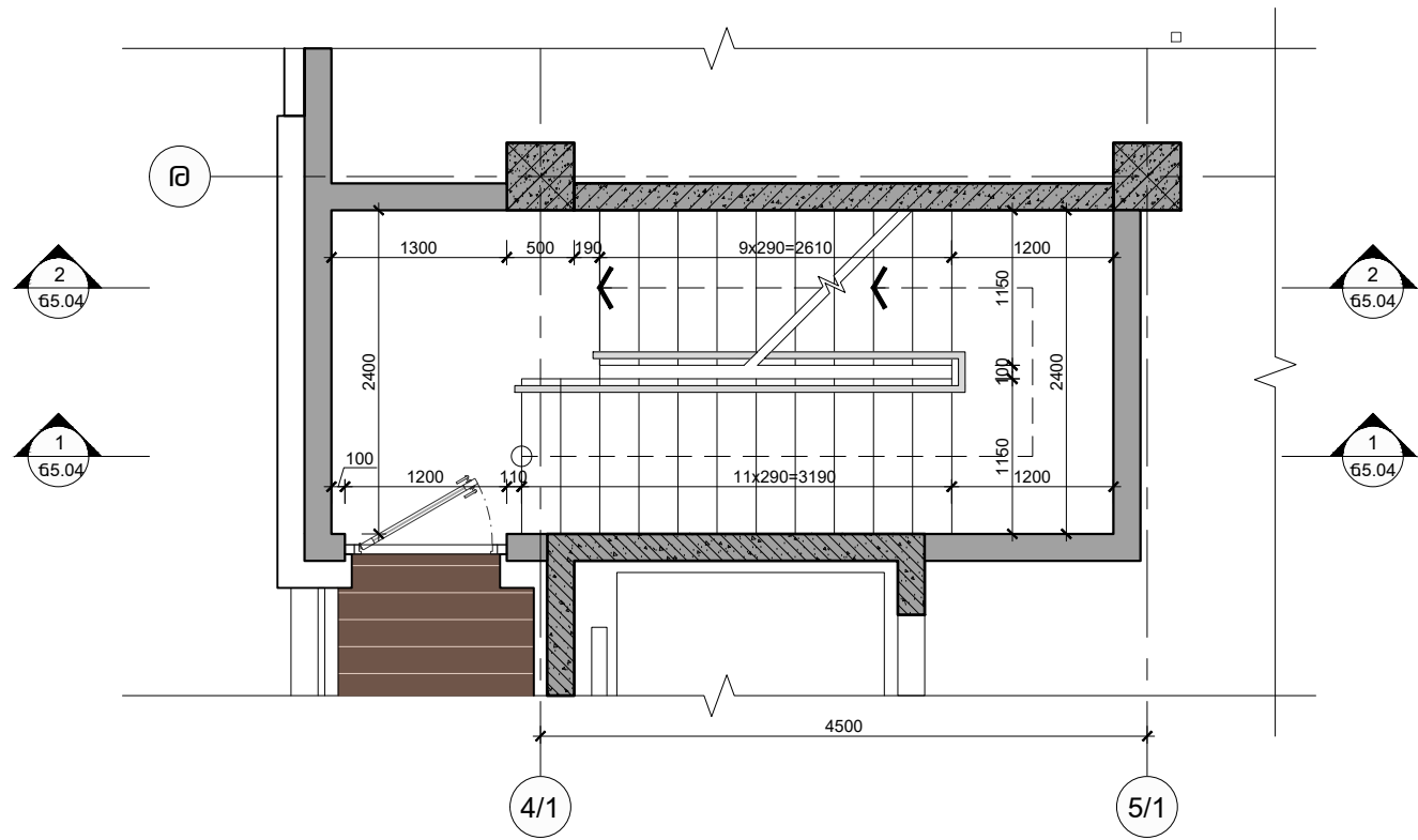
ԱՍՏԻՃԱՆԱՎԱՆՂԱԿ 2, ԴՐՎԱԳ 4 (8-ՐԴ ՀԱՐԿԻ ՀԱՏԱԿԱԳԻԾ) Մ 1:50
