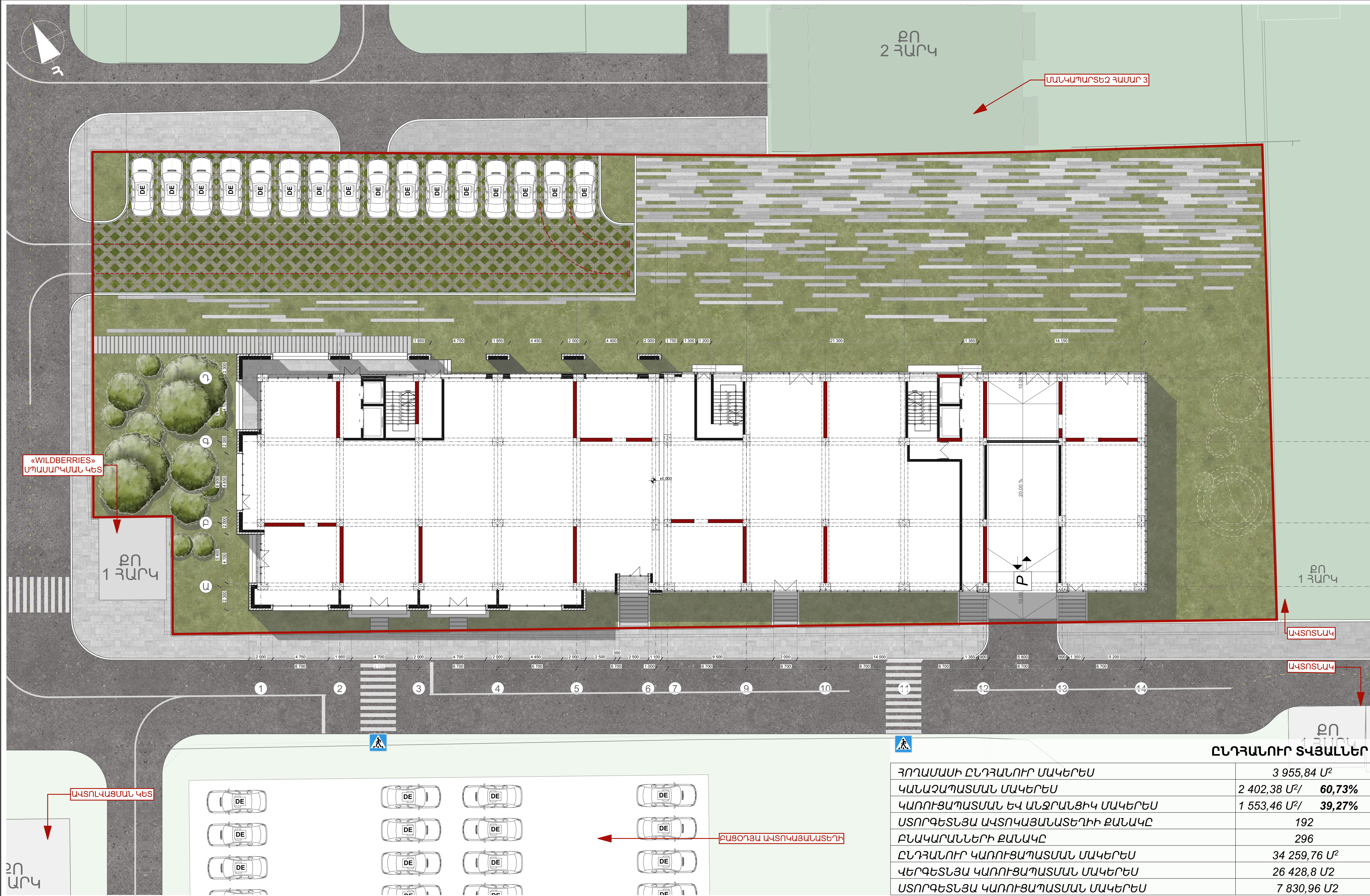
ՔԼԽԱՎՈՐ ՀԱՏԱԿԱԳԻԾ Մ 1:200
