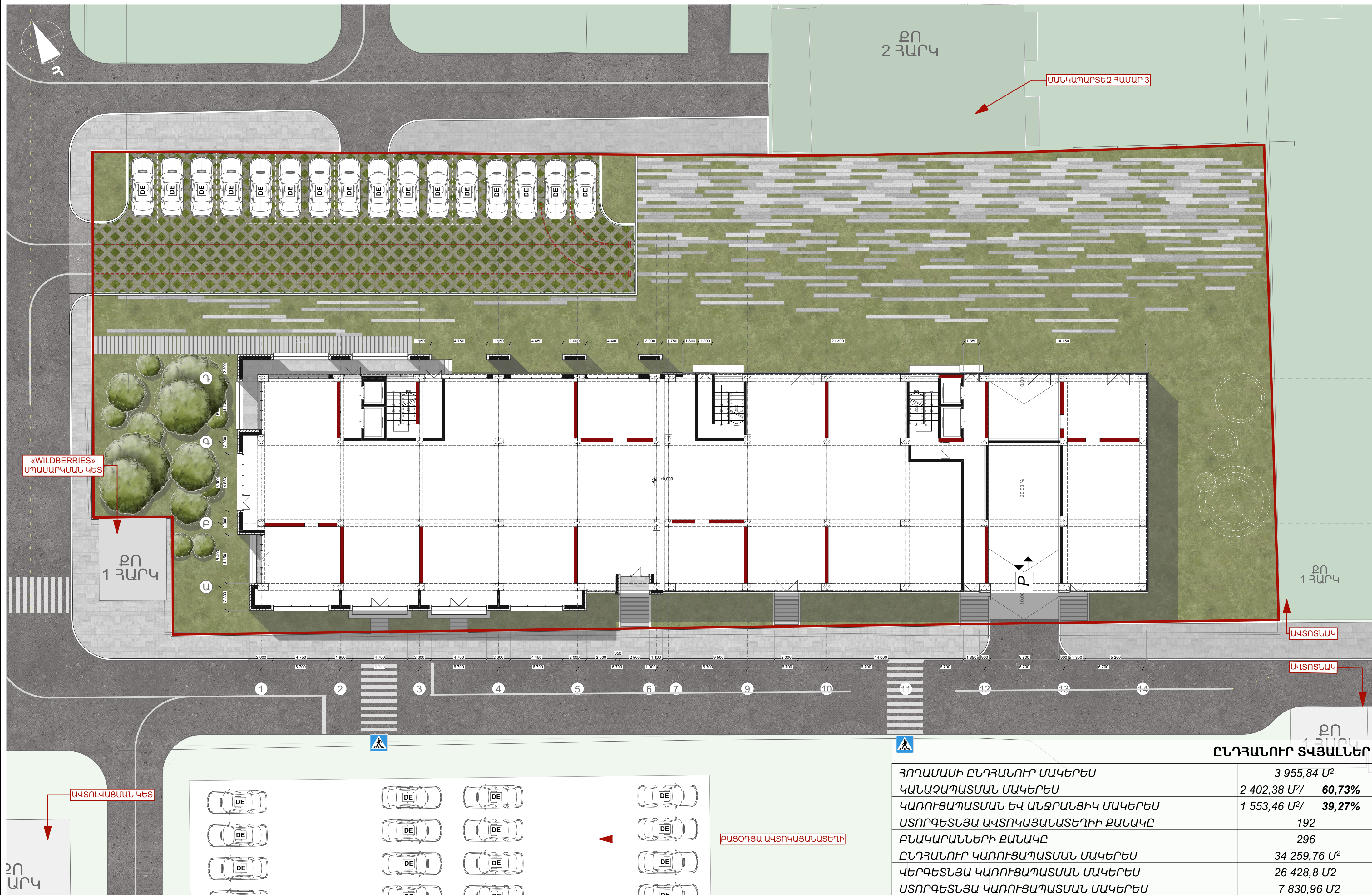
ՓԼԱՆԱՎՈՐ ՀԱՏԱԿԱԳԻԾ Մ 1:200
